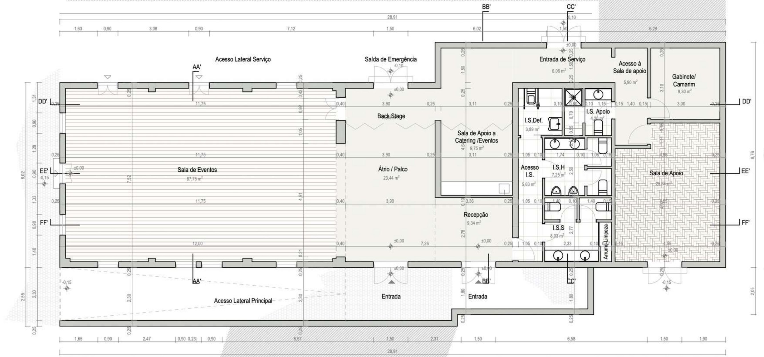
PLANTA PISO TÉRREO
